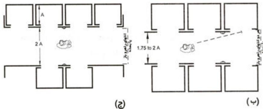
شکل ۱۵-۲-۱-۴ (ب) فضاهای انتظار در راهروهای مقابل آسانسورها
