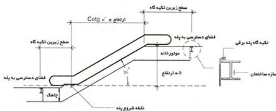
شکل ۱-۲-۳-۱۵ طرح کلی پله برقی
