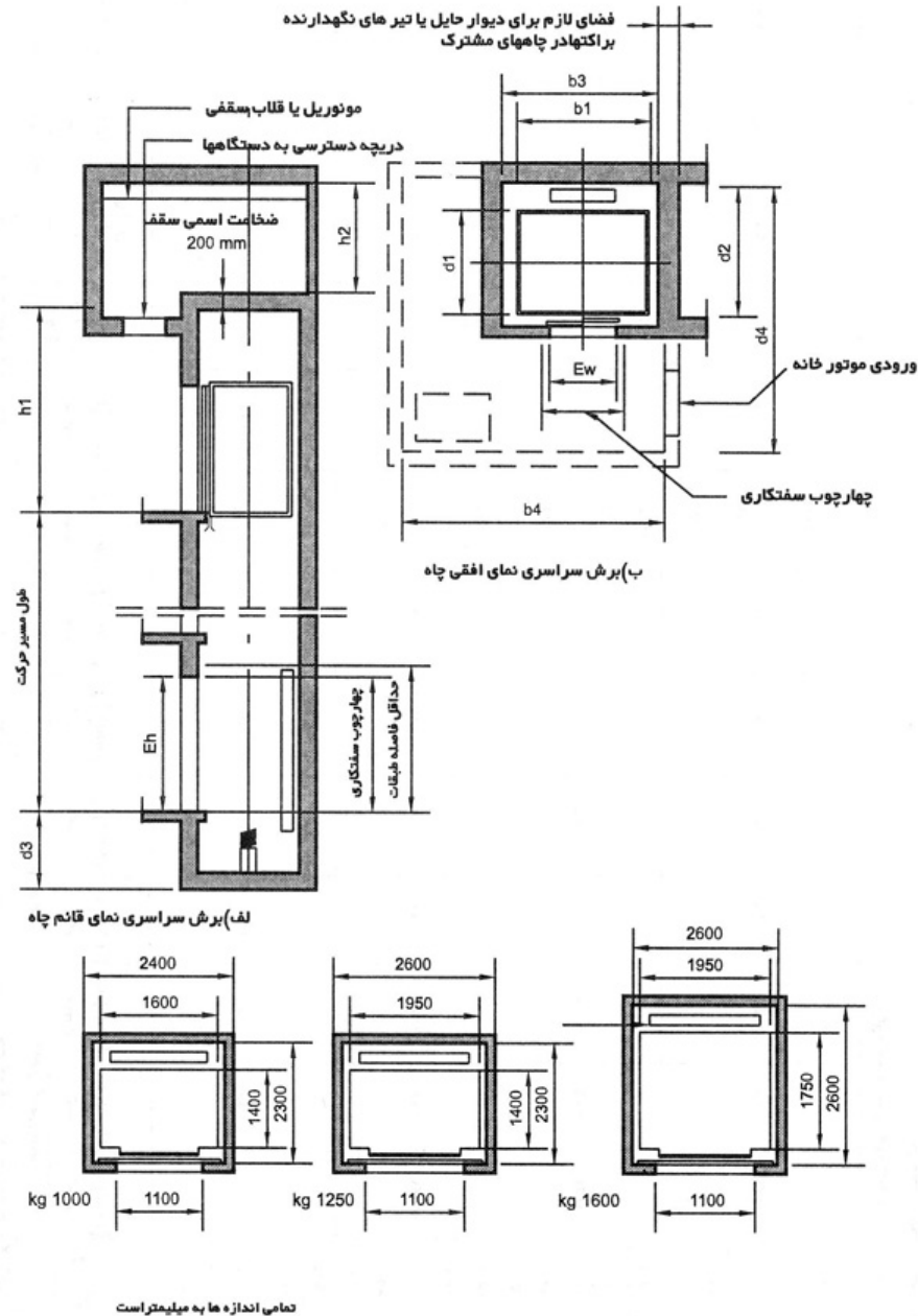
شکل ۵- طرح اولیه معماری آسانسور های الکتریکی مسافری بانرد ز یاد
