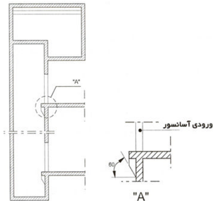
شکل ۴-۲-۲-۲-۱۵ سطح داخلی دیواره چاه در سمت ورودی طبقات
