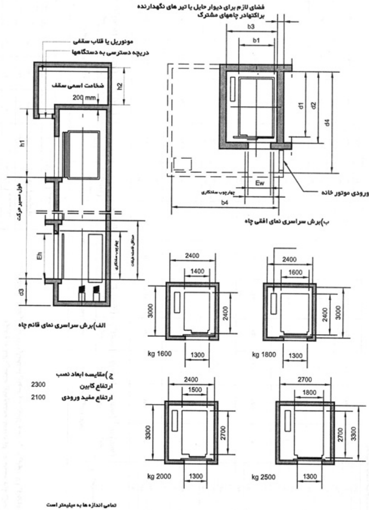
شکل ۶- طرح اولیه معماری آسانسورهای الکتریکی حمل تخت بیمار و مسافر
