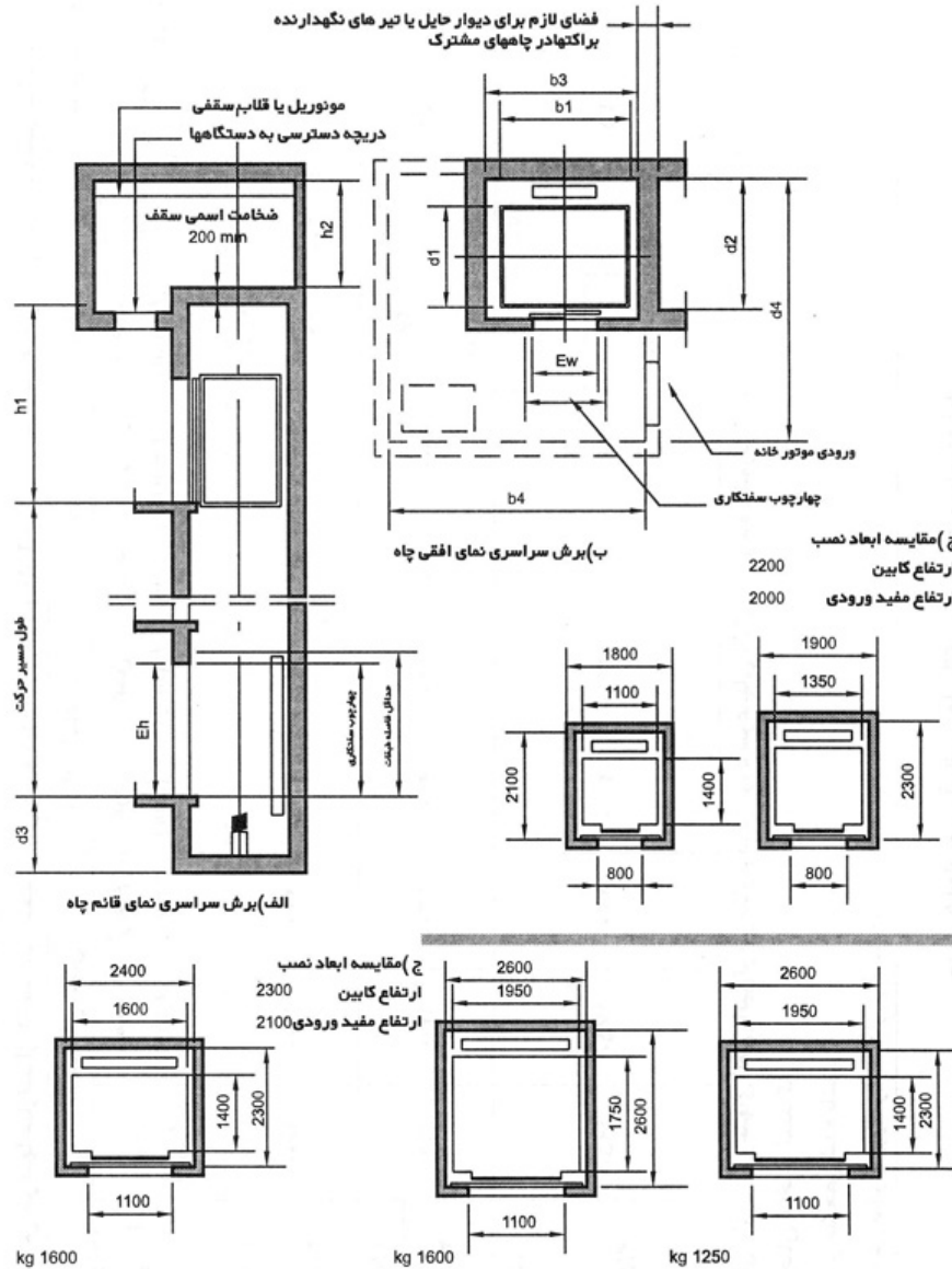
شکل ۴- طرح اولیه معماری آسانسورهای الکتریکی مسافری با کاربرد عمومی
