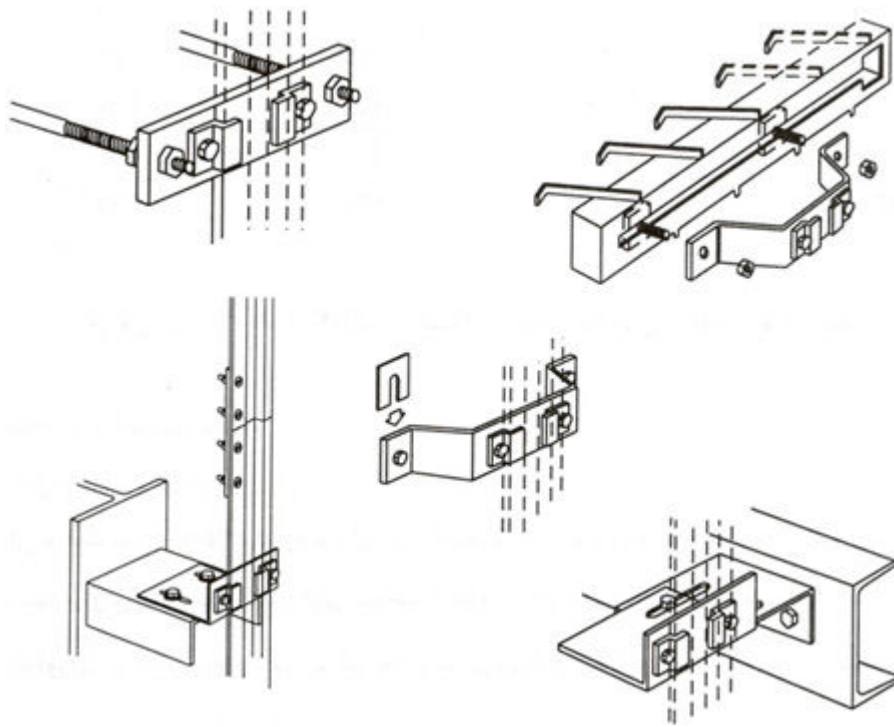
۱-۲-۲-۲-۱۵ انواع براکت و نحوه اتصال به سازه های فلزی و بتنی
