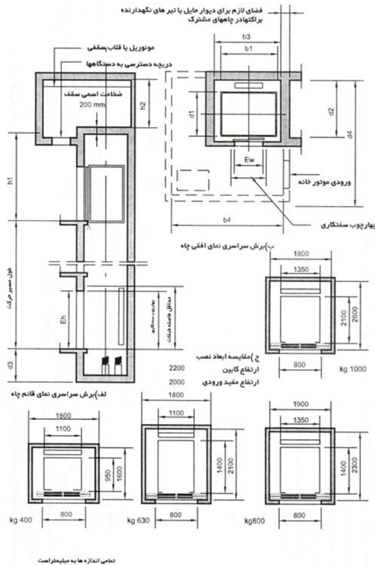
شکل ۱-۲ طرح اولیه معماری آسانسورهای الکتریکی ساختمان های مسکونی
