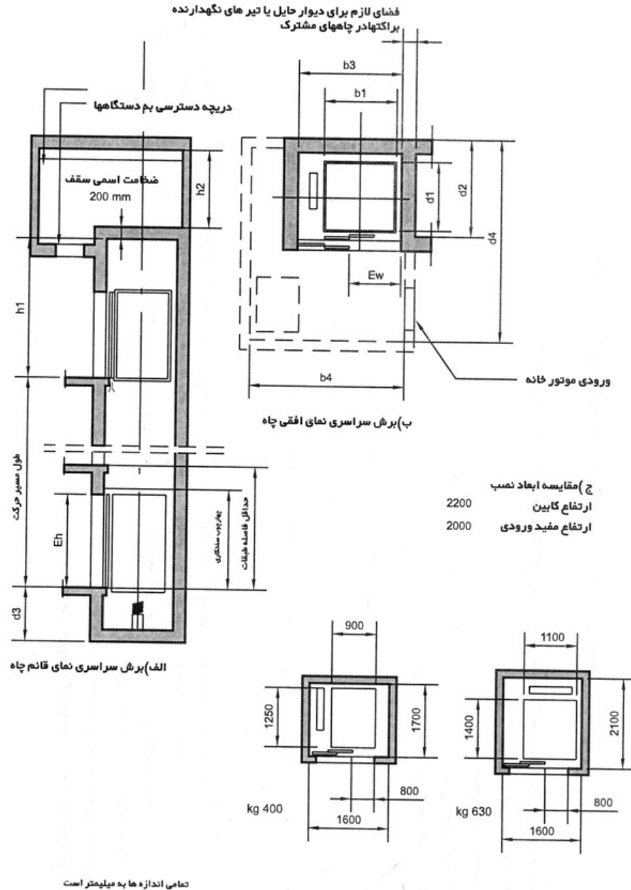
شکل ۲-۳- طرح اولیه معماری آسانسورهای الکتریکی مسافری با تردد موردی
